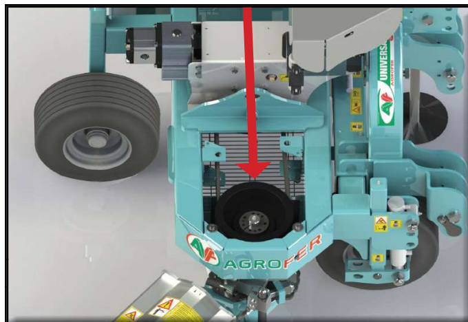
TRASMISSIONE MECCANICA A CINGHIA
